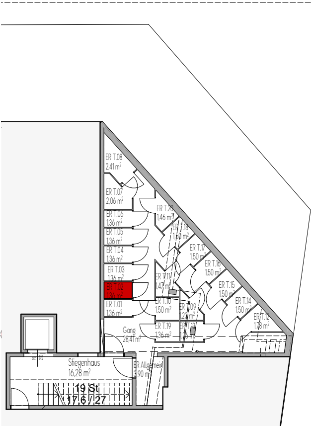
Tiefgeschoß - Einlagerungsraum
