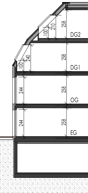
Konzept Fassadenschnitt
