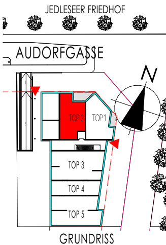
Tiefgeschoß - Einlagerungsraum
