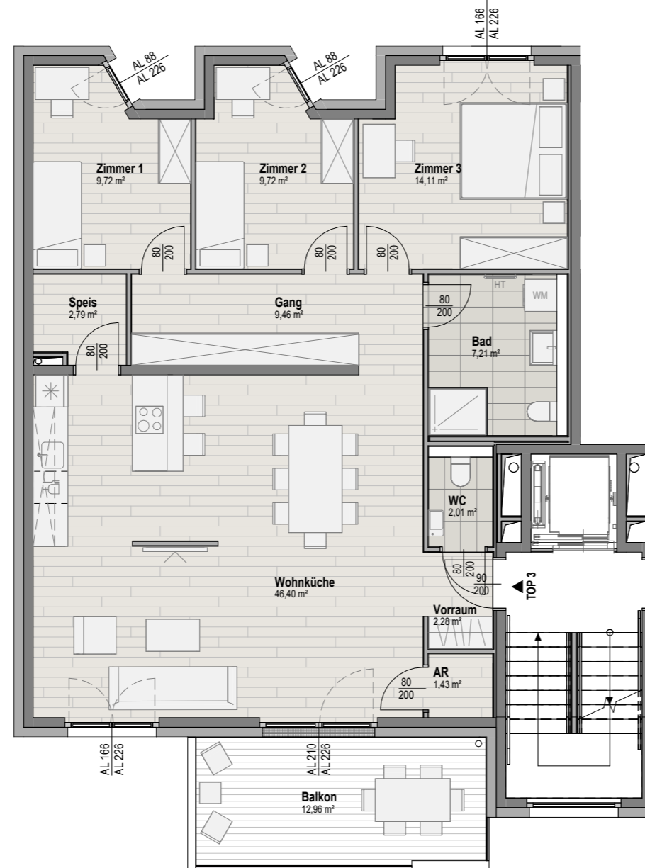
GRUNDRISS WOHNUNG
